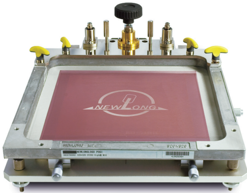
HP-320 (卓上型手刷りスクリーン印刷機)
