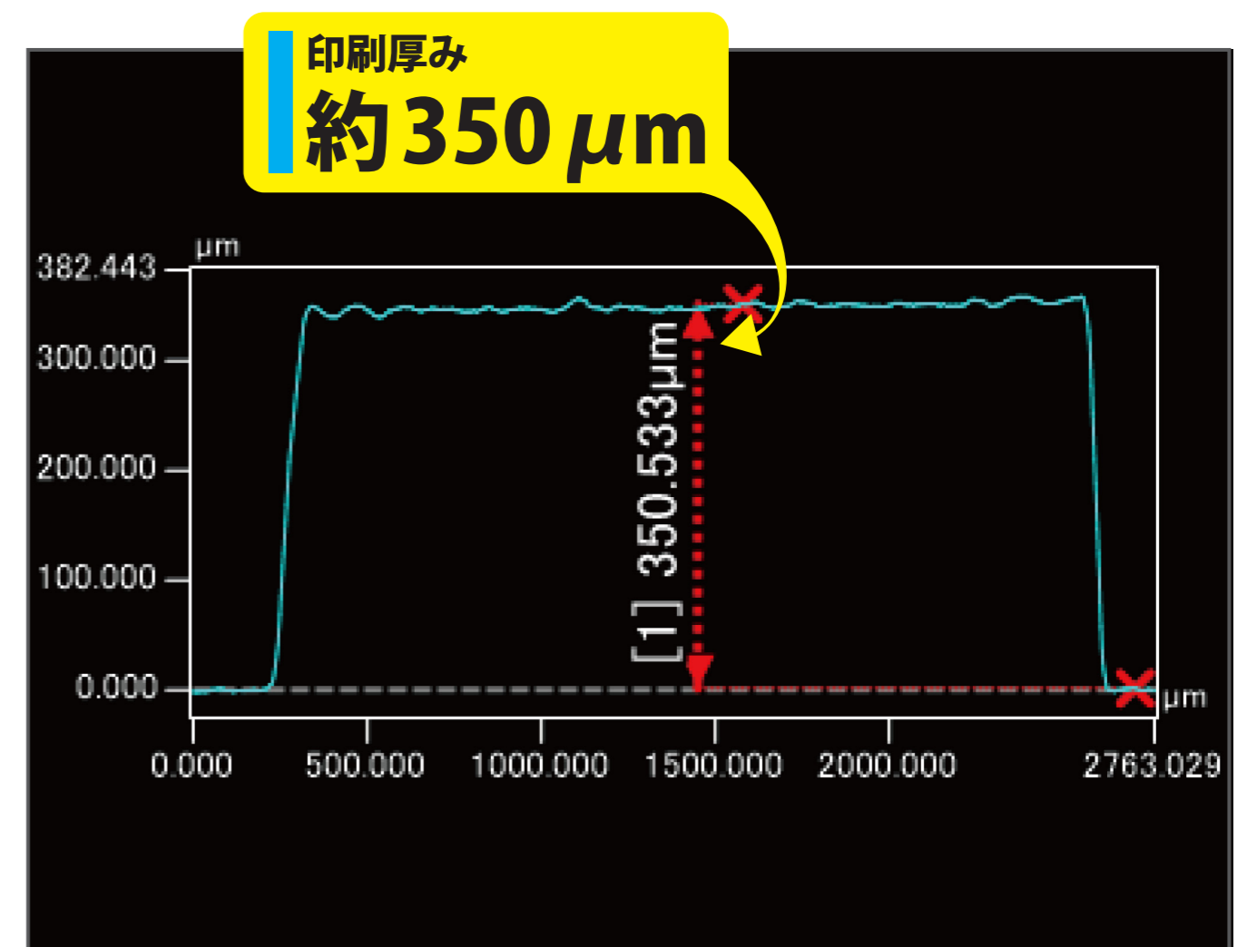
厚み測定結果
