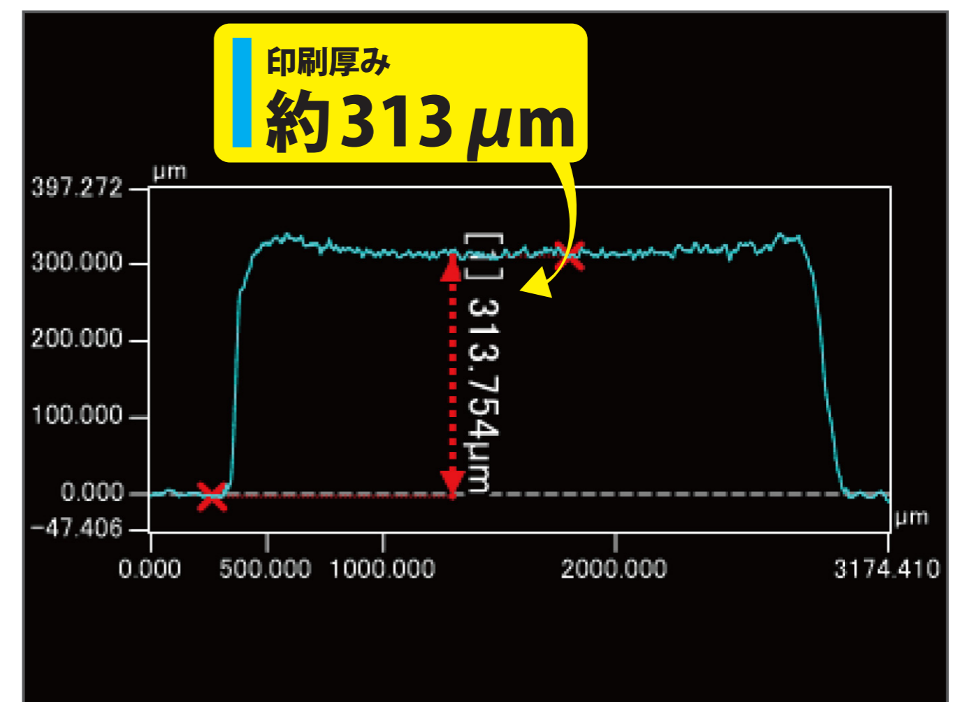
厚み測定結果
